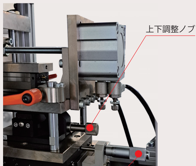
前後調整マイクロメーター
